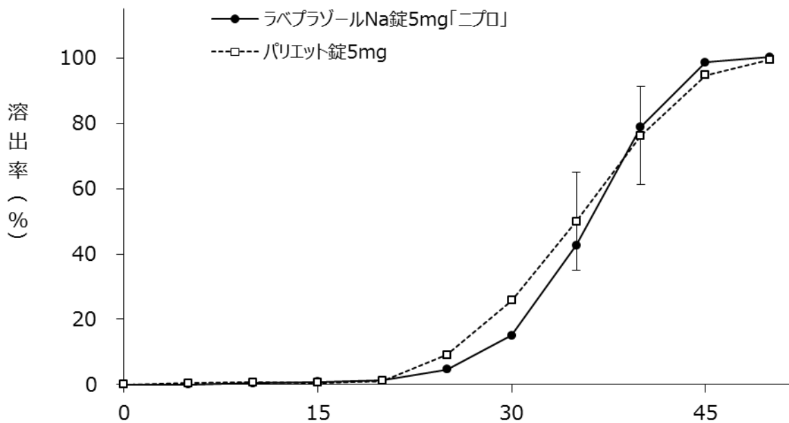
図4 試験液：pH 6.0 (100 rpm)
